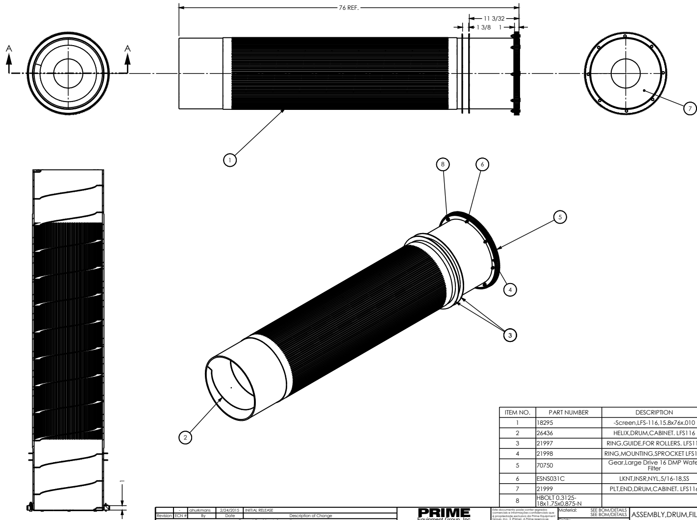
SECTION A-A SCALE 1 : 8
